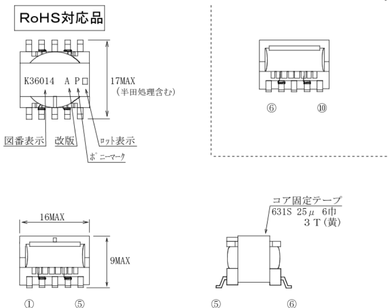
外形図
