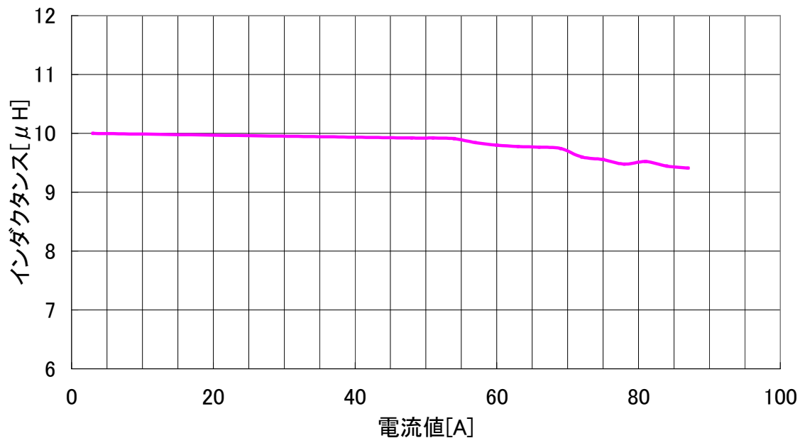
P009-306 直流重畳特性(換算値(実験値))
