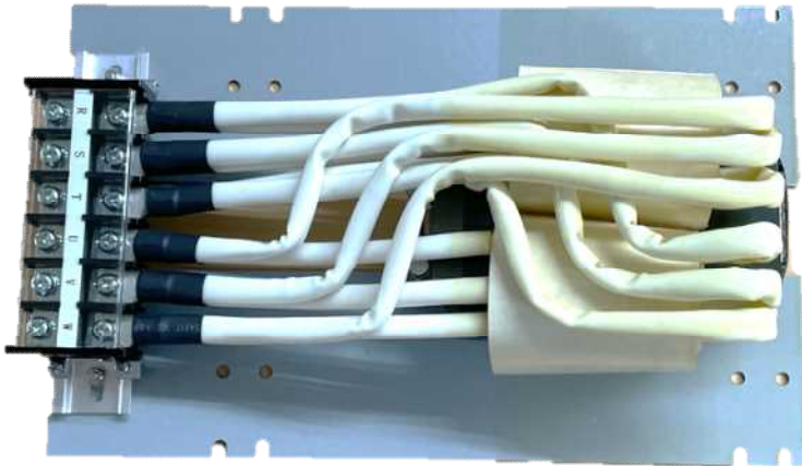
P022-630 W180 × D130 × H140 インダクタンス 1mH 電流値(RMS) 40A
